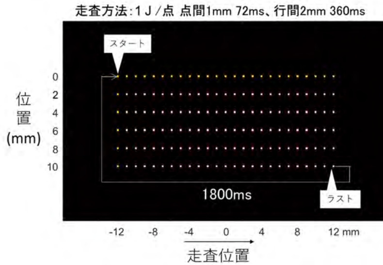
図A 6 面状照射パターン (行間 2mm、戻り 1800ms)
