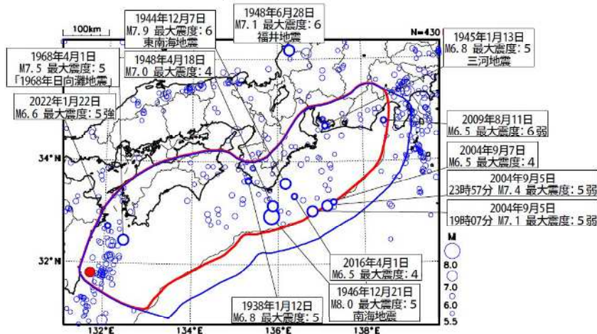
震央分布図
